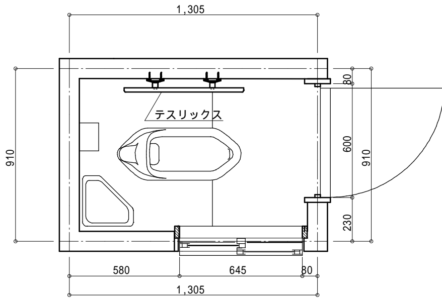
平面図
