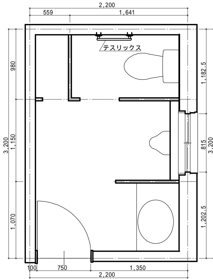
平面図
