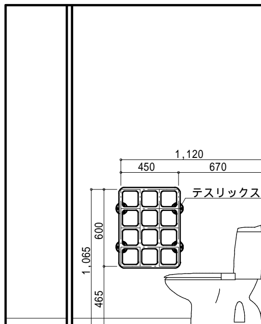
テスリックス 取付側展開図
