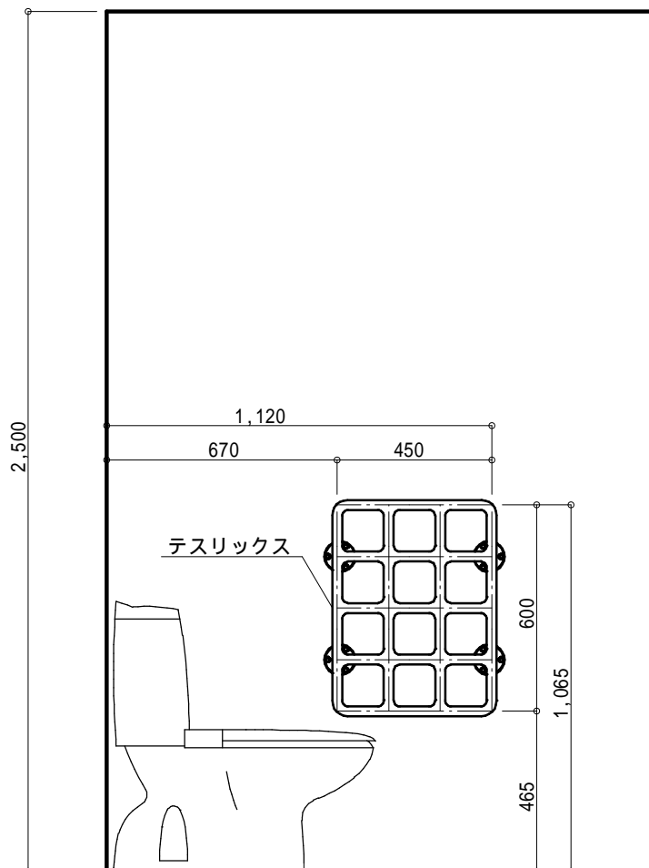
テスリックス 取付側展開図
