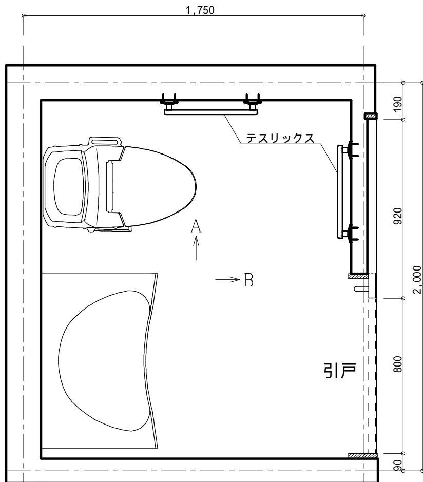
平面図
