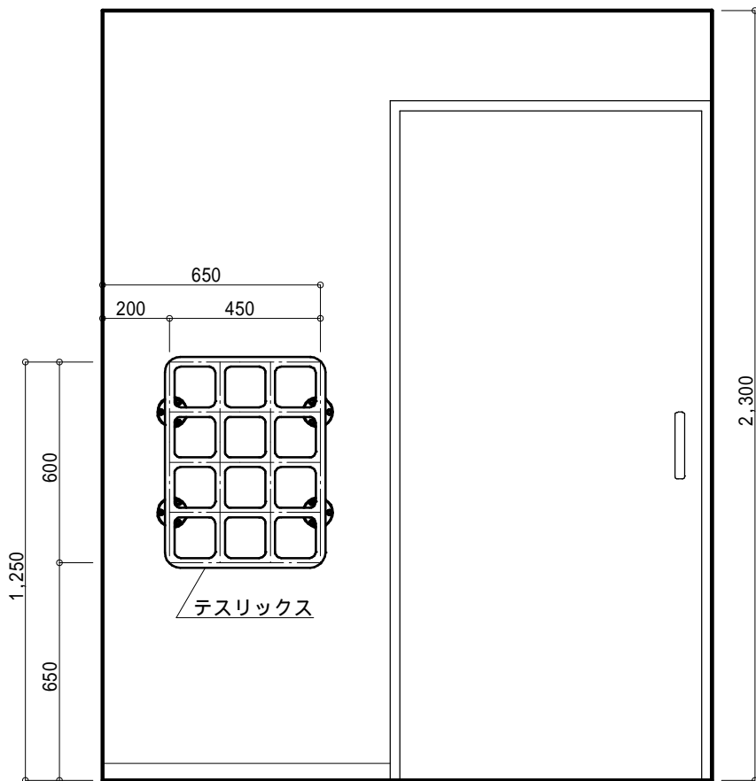
B面
