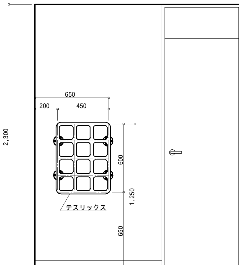
テストリックス 取付側展開図
