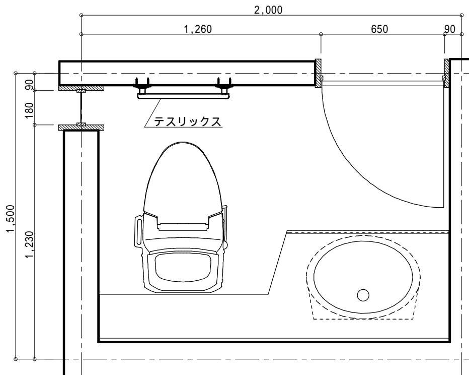
平面図
