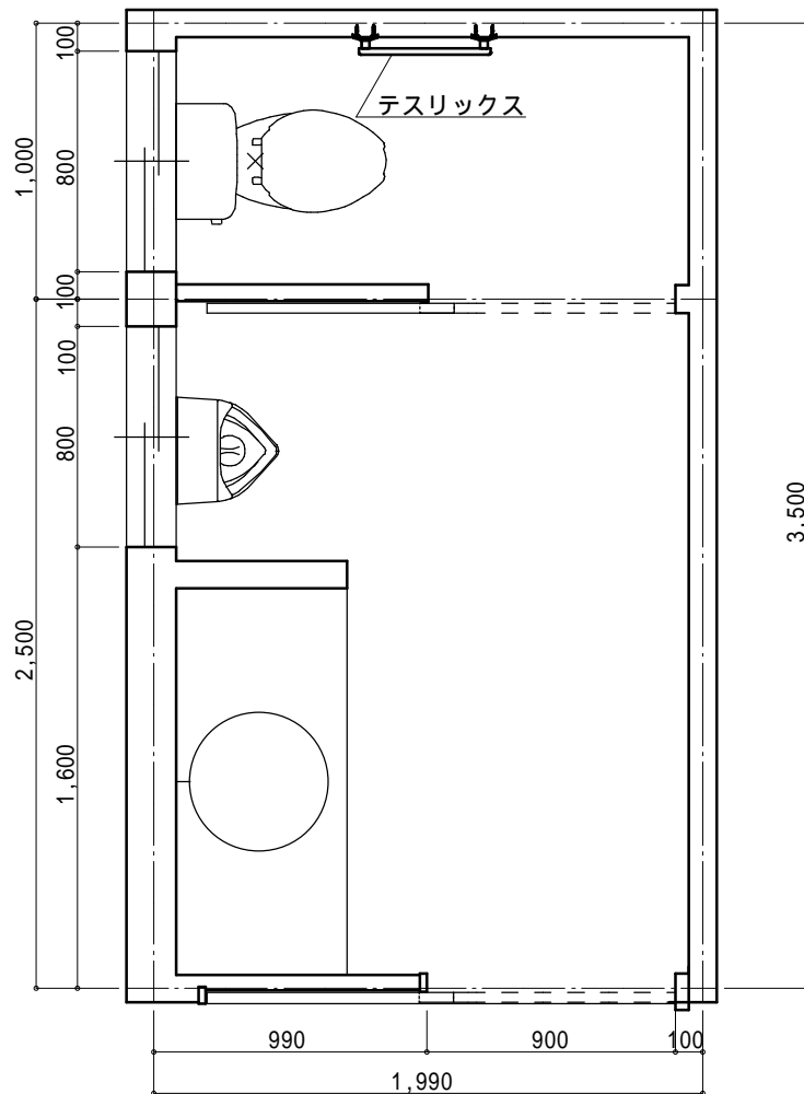
平面図
