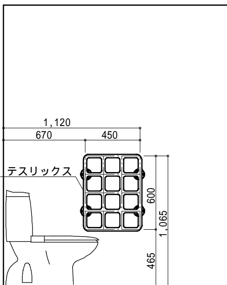
テスリックス 取付側展開図
