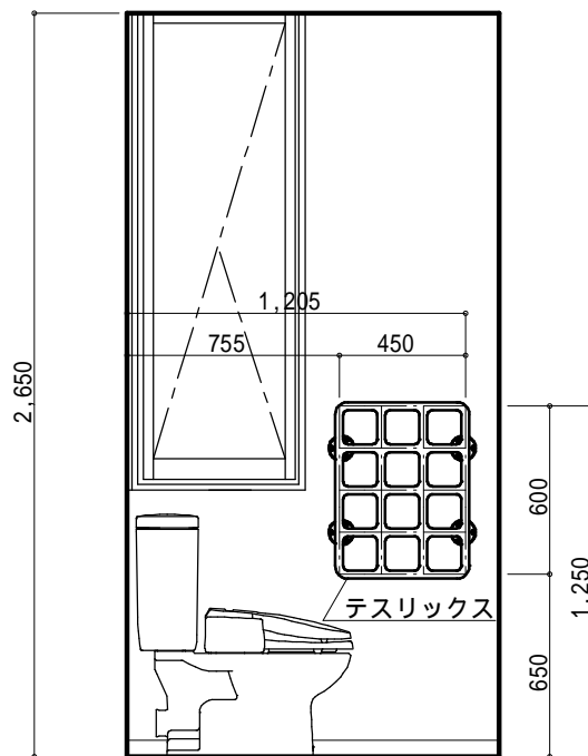
テスリックス 取付側展開図
