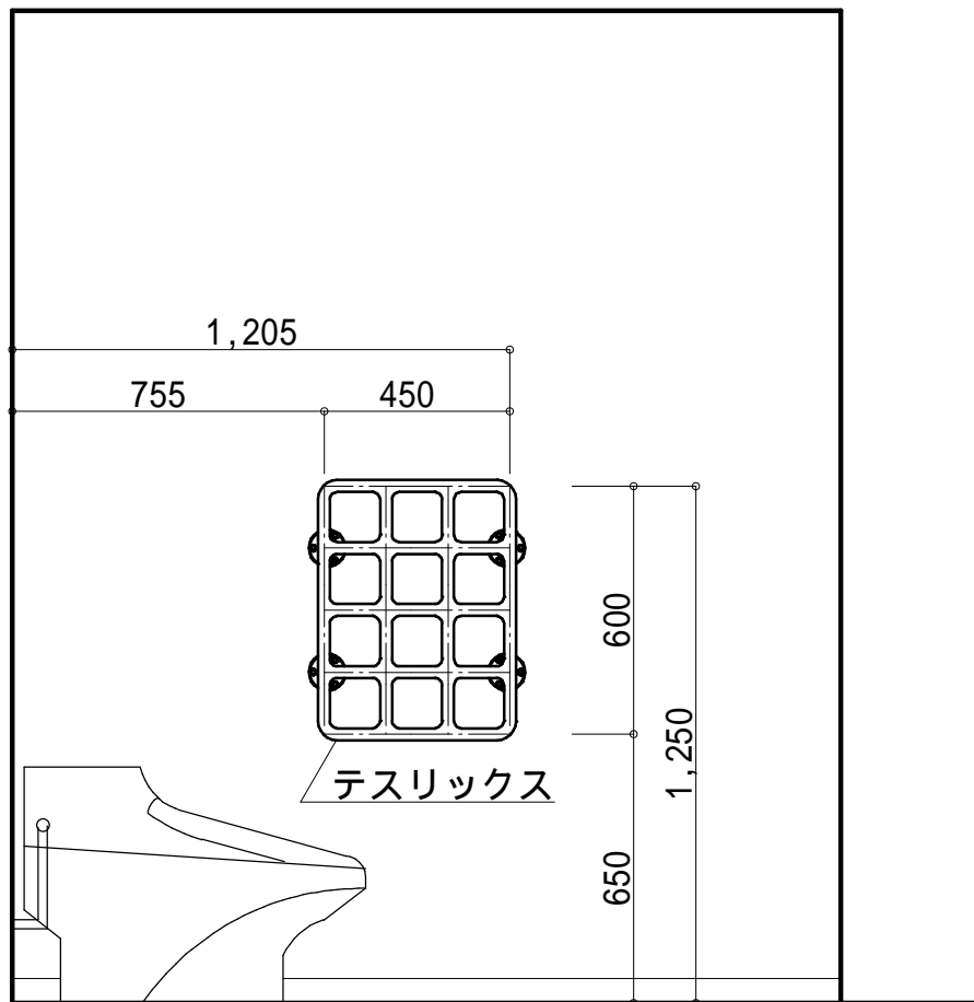
テスリックス 取付側展開図
