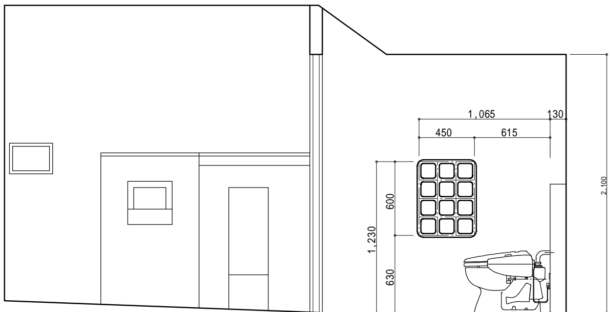
テスリックス 取付側展開図
