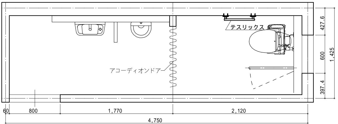
平面図
