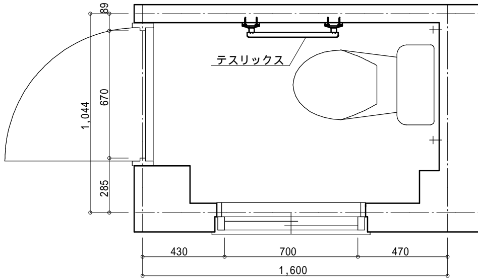
平面図
