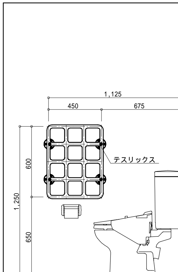
テスリックス 取付側展開図
