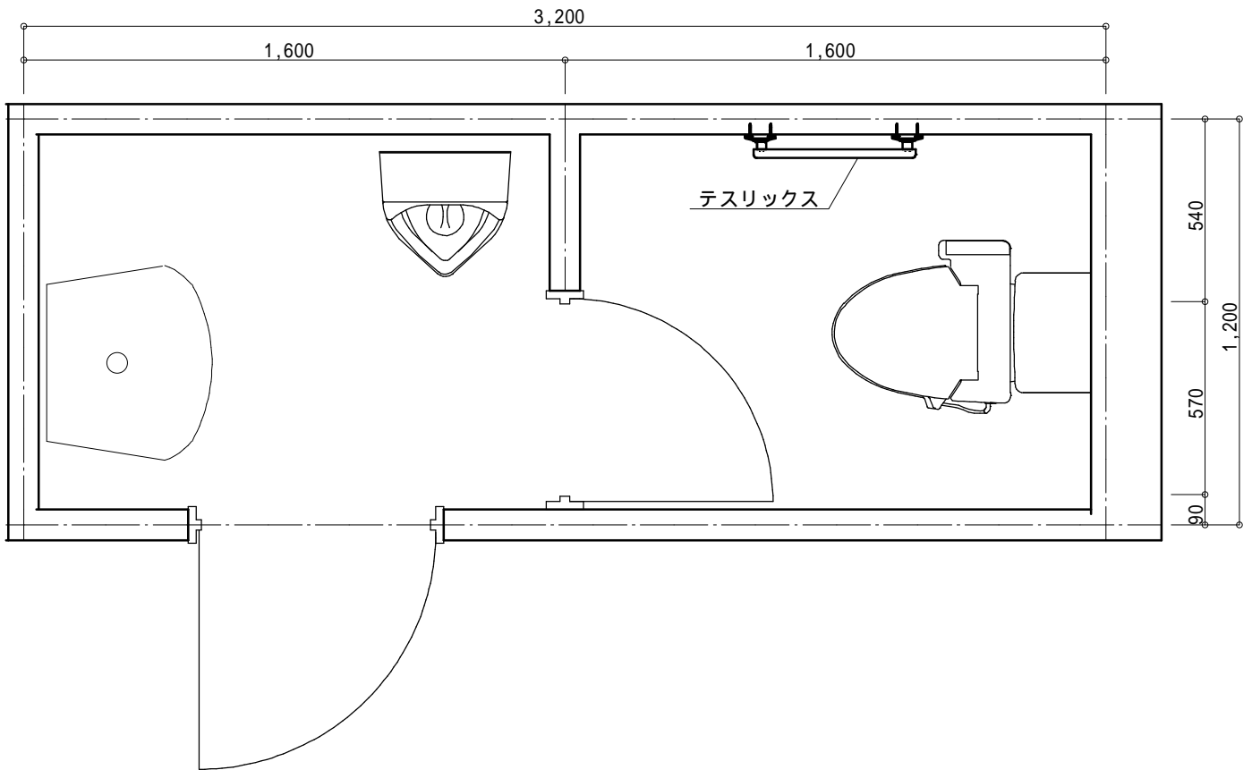
平面図
