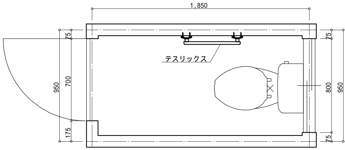
平面図
