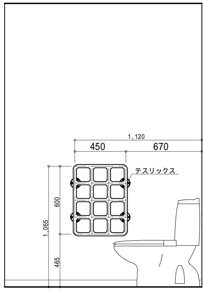
テスリック 取付側展開図
