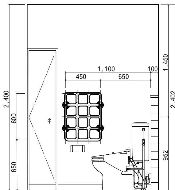
テスリックス 取付側展開図
