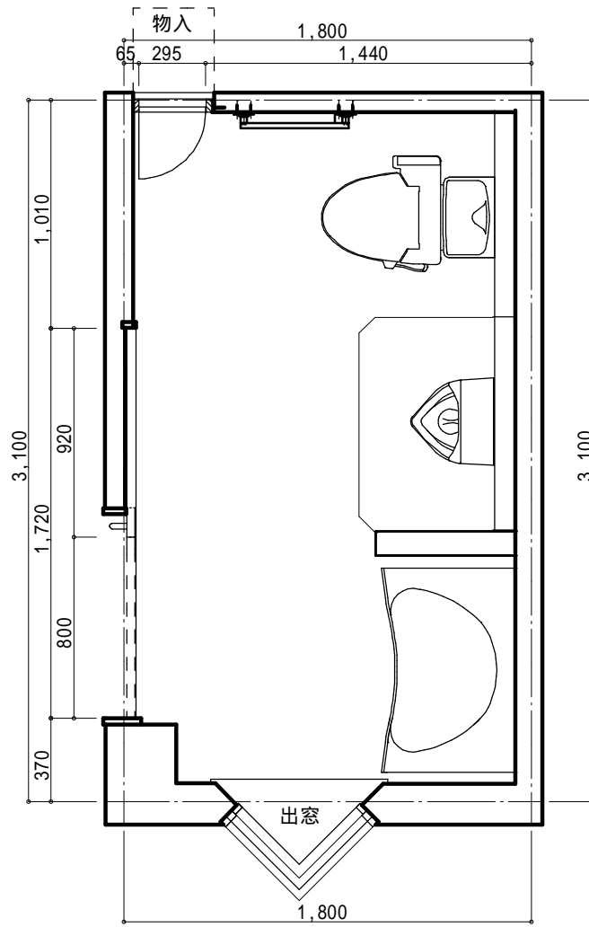
平面図
