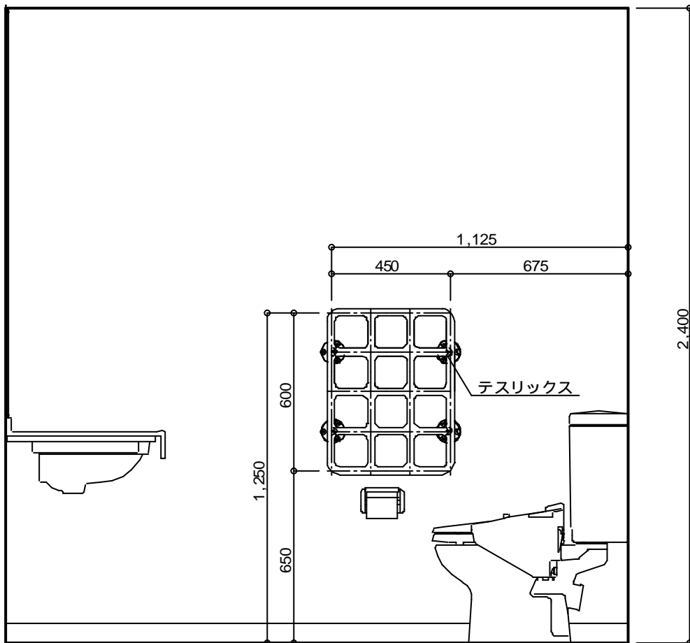
テスリックス 取付側展開図
