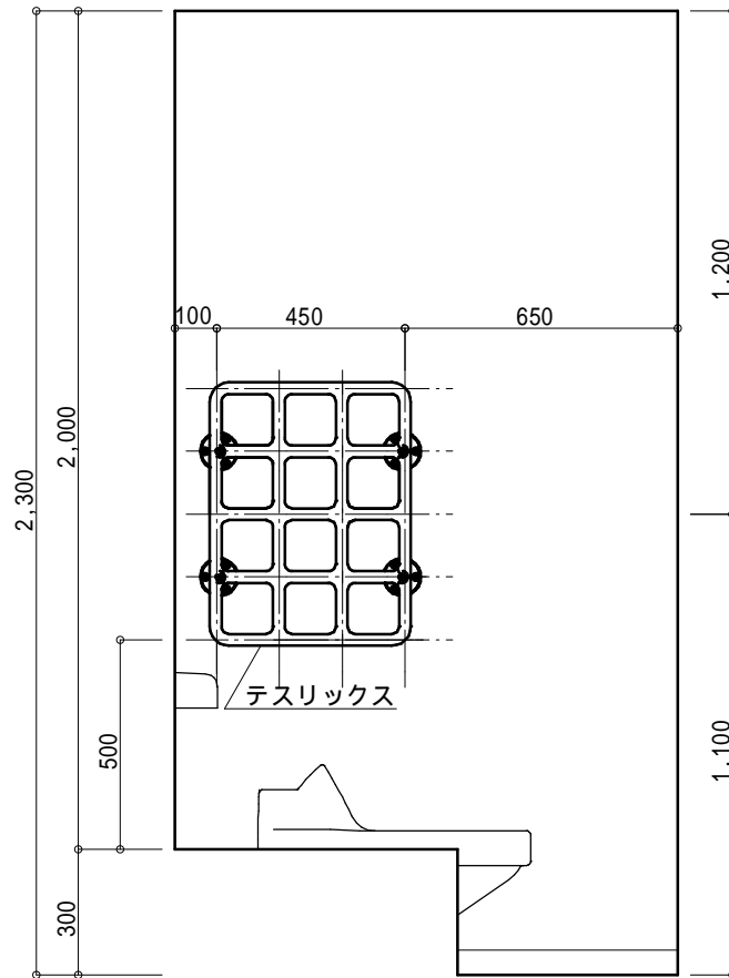
テスリックス 取付側展開図
